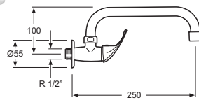
Ref. 3122201-1 Cromo Fregadero pared caño alto tubo 1 sola agua
